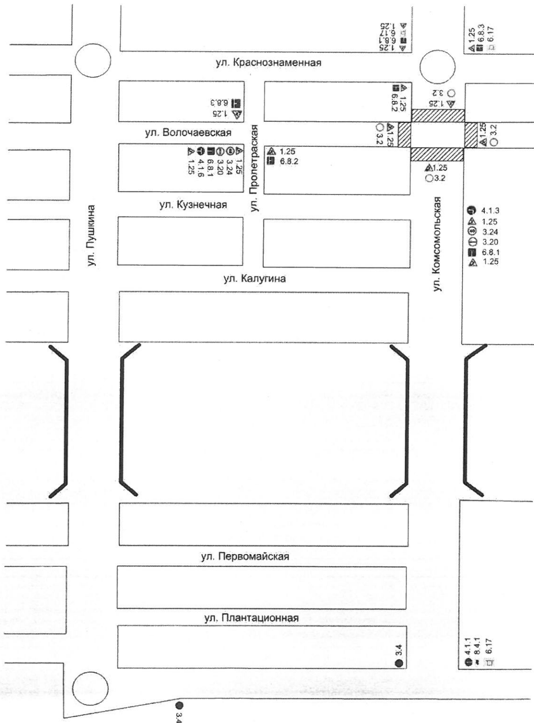
Схема ограждений места производства работ на перекрестке ул. Волочаевская – ул. Комсомольская
